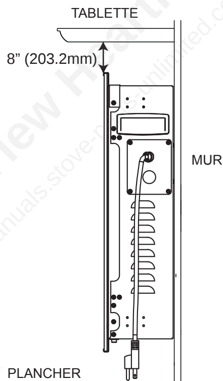
VUE DU CÔTÉ
