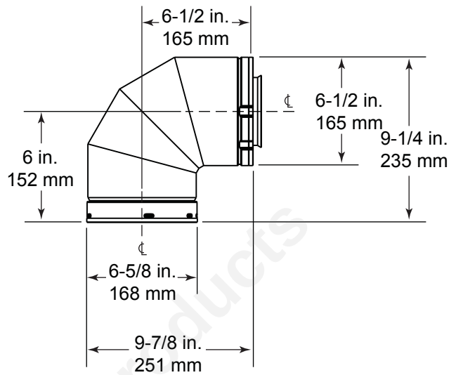
SLP90- 90° Elbow
