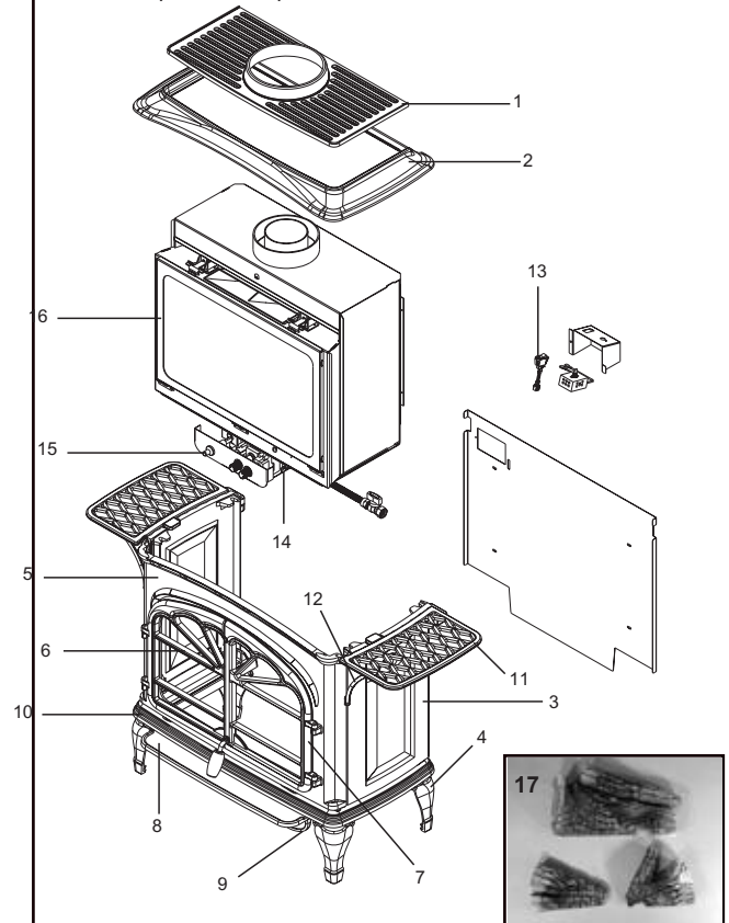
TIARA II EXPLODED DRAWING /Vue éclatée des pièces
