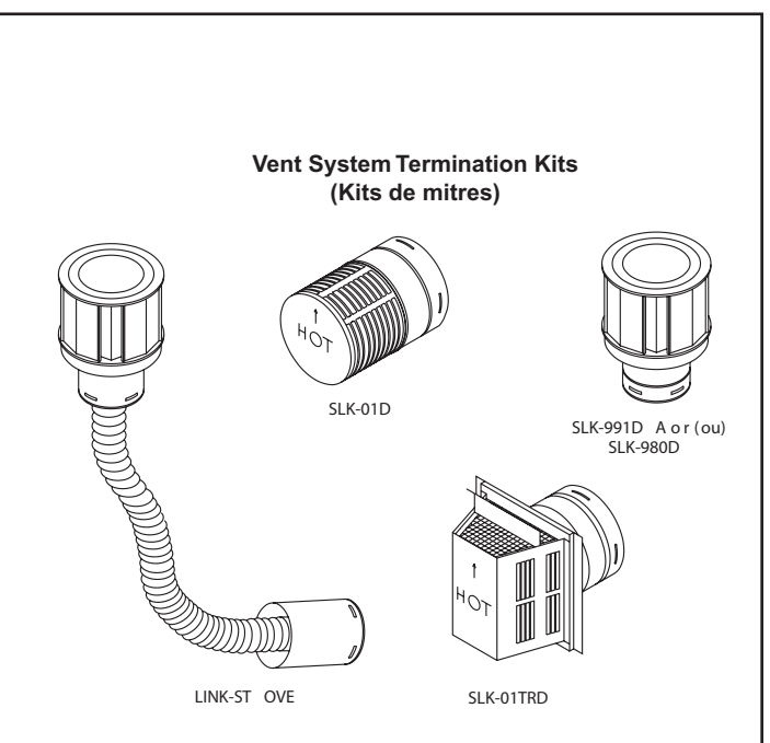
◆ Figure 4. Éléments du système de ventilation et mitres ◆
