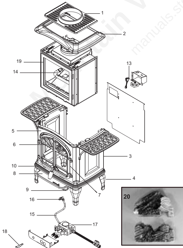
TIARA I EXPLODED DRAWING/Vue éclatée des pièces
