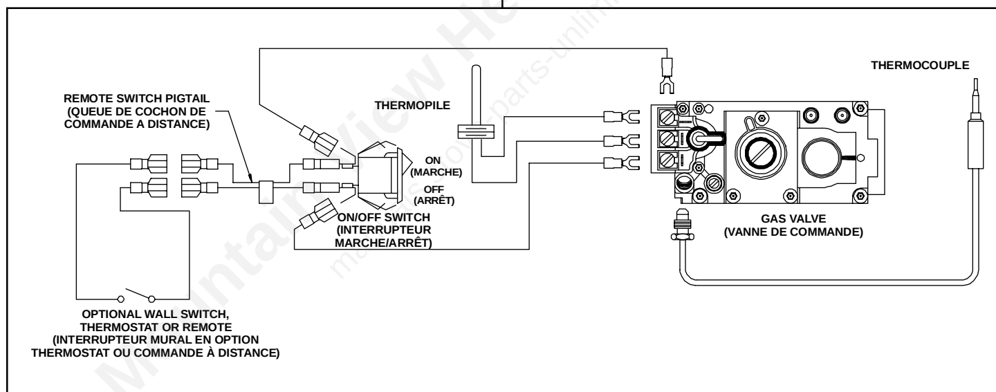
Figure 24. Schéma de câblage de l'allumage par veilleuse
