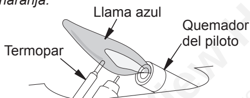
Figura 22 - Patrón correcto de la llama del piloto
