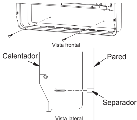
Figura 12 - Instalación de los tornillos de montaje inferiores
