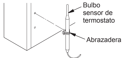
Figura 5 - Instalación del bulbo sensor de termostato
