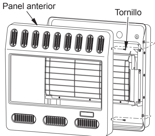
Figura 7 - Desmontaje del panel anterior del calentador
