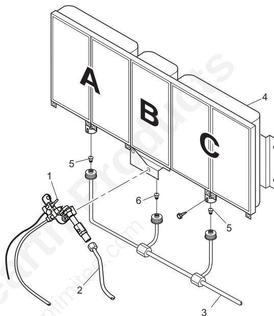
Conjunto de quemador LCR26PT, LCR30NT, HDR26PT y HDR30NT
