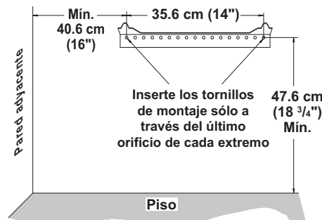
Calentador con 5 placas
