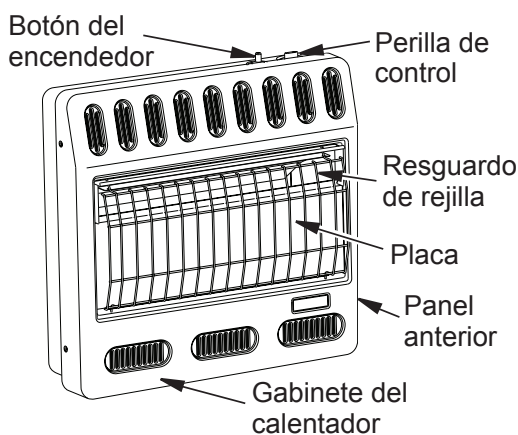
Figura 1 - Calentador de gas sin ventilación
