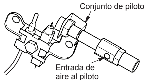
Figura 26 - Entrada de aire del piloto
