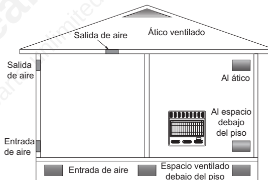
Figura 3 - Aire del exterior para ventilación
