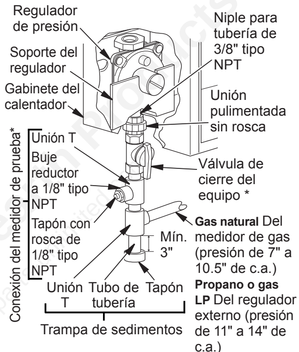
Figura 14 - Regulador externo con la ventila apuntando hacia abajo
