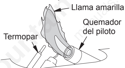
Figura 23 - Patrón incorrecto de la llama del piloto
