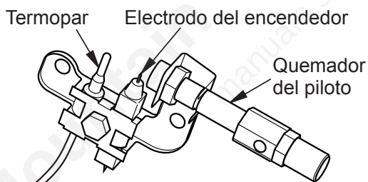
Figura 20 - Piloto
