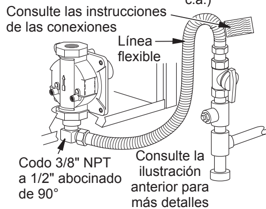
Figura 15 - Conexión de gas
