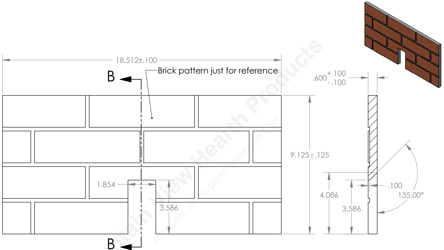
SECTION B-B SCALE 1 : 3
