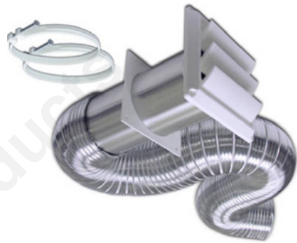
Installation du «kit de ventilation de la sécheuse»
