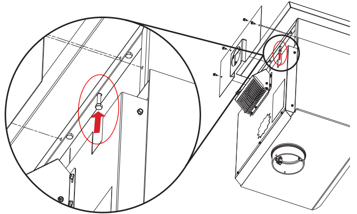
Illustration: Fixation du réchauffeur au plancher.
