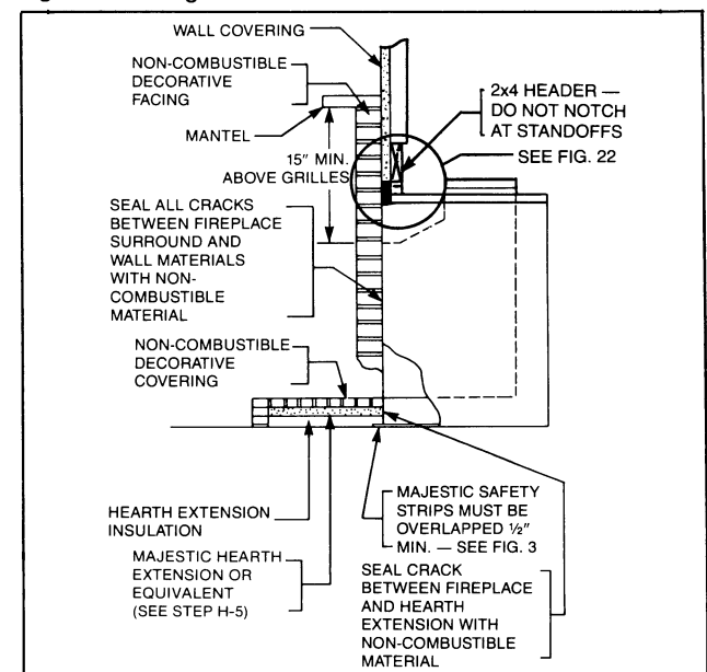
Fig. 27. Sealing detail.
