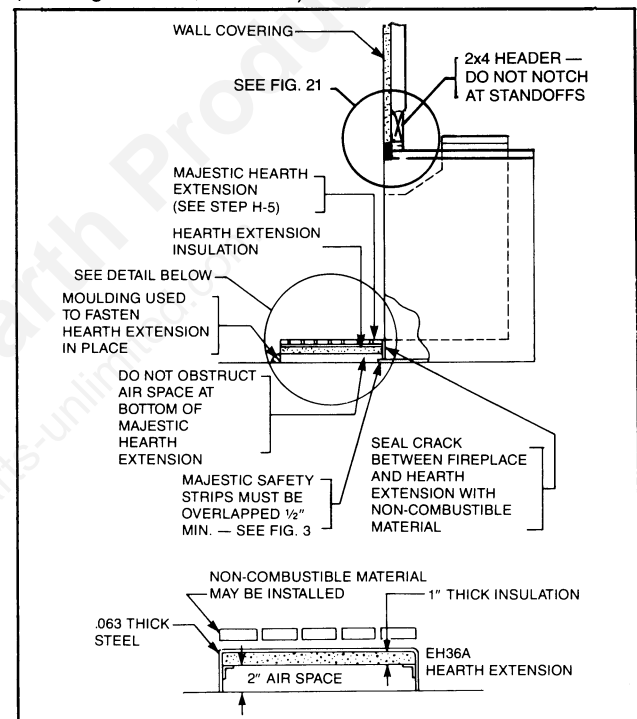
Fig. 26. Sealing detail.
