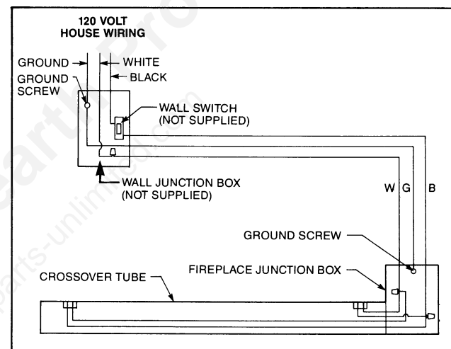
Fig. 15. Wiring diagram.
