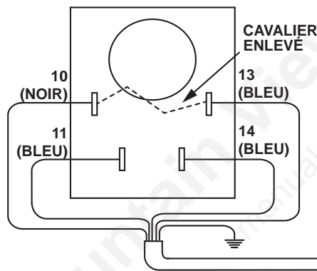
INTERRUPTEUR DE VITESSE DE LA SOUFFLERIE ET DE SURCHAUFFE DE LA FOURNAISE À L'HUILE
