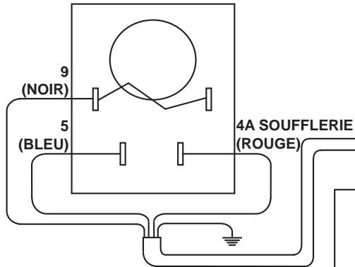
INTERRUPTEUR DE VITESSE DE LA SOUFFLERIE ET DE SURCHAUFFE DE LA FOURNAISE À BOIS
