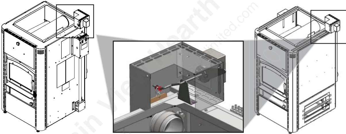
PLAQUE DU VOLET D'AIR
