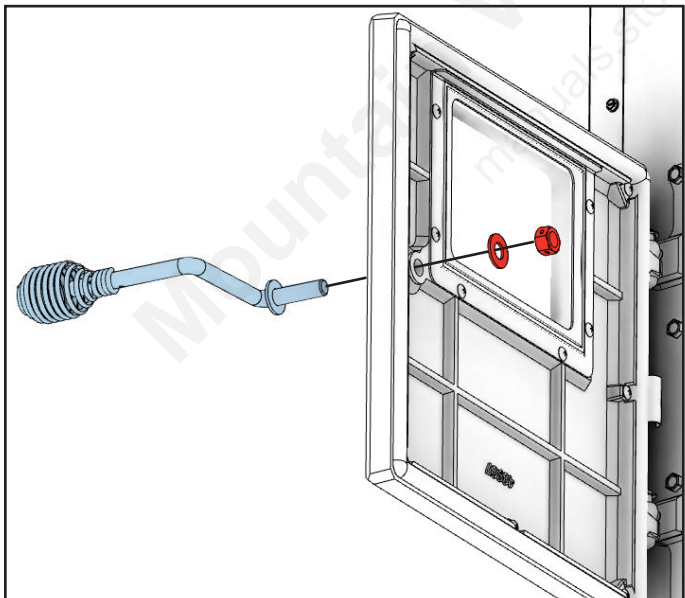
Utilisez un (1) écrou et une (1) rondelle pour fixer la poignée au poêle comme indiqué. Remarque : Ajustez la poignée selon les besoins pour assurer une bonne étanchéité.
