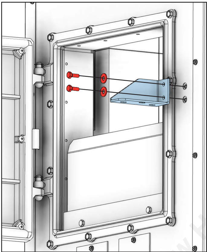
Utilisez deux (2) boulons 1/4-20 x 3/4 et deux (2) rondelles pour fixer le loquet à l'unité.
